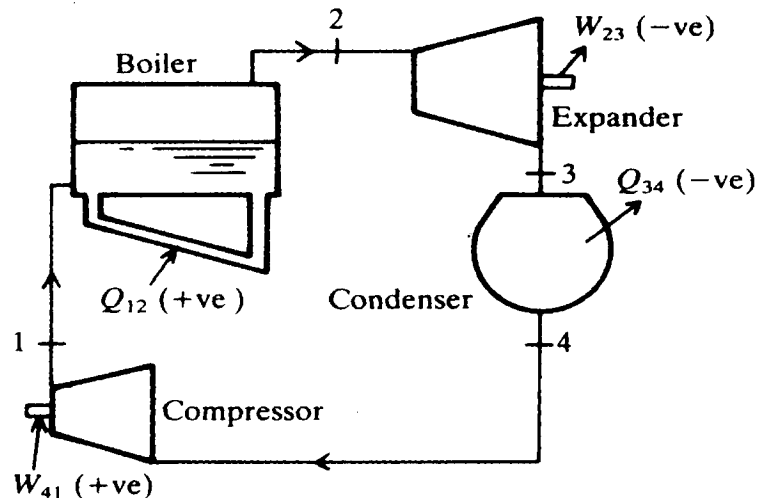
Fig Q5: Carnot Vapour Cycle
