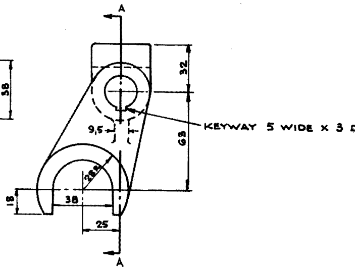
END ELEVATION
